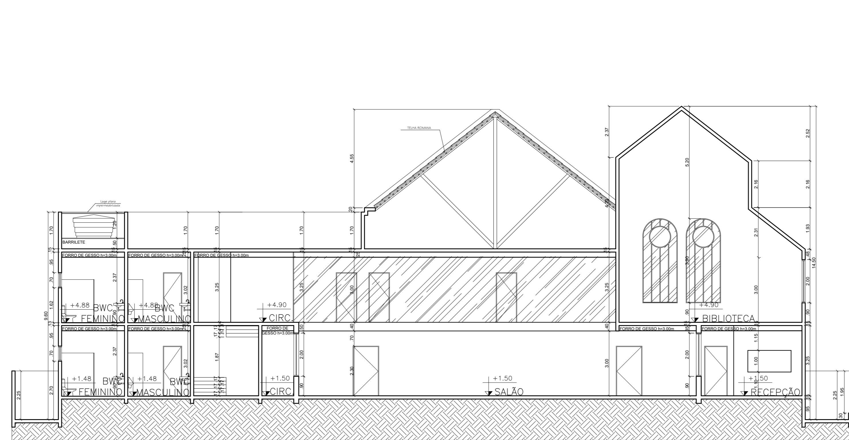
05 CORTE AA' ESCALA 1:100
