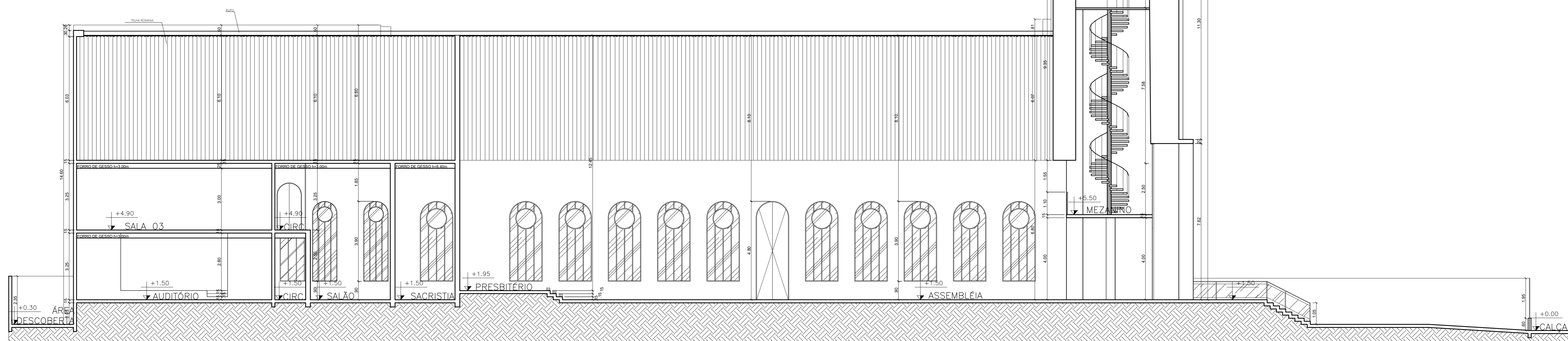
06 CORTE BB' ESCALA 1:100
